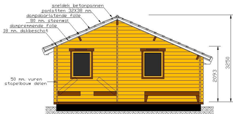
voorgevel
