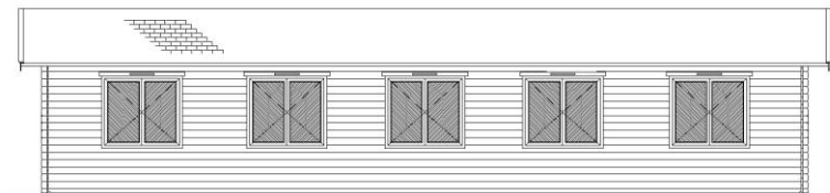
linkerzijgevel
