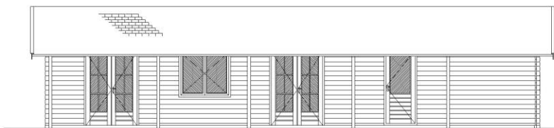
rechterzijgevel
